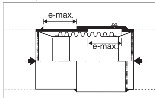
E-karmantyú \varnothing 168,3-610 mm
